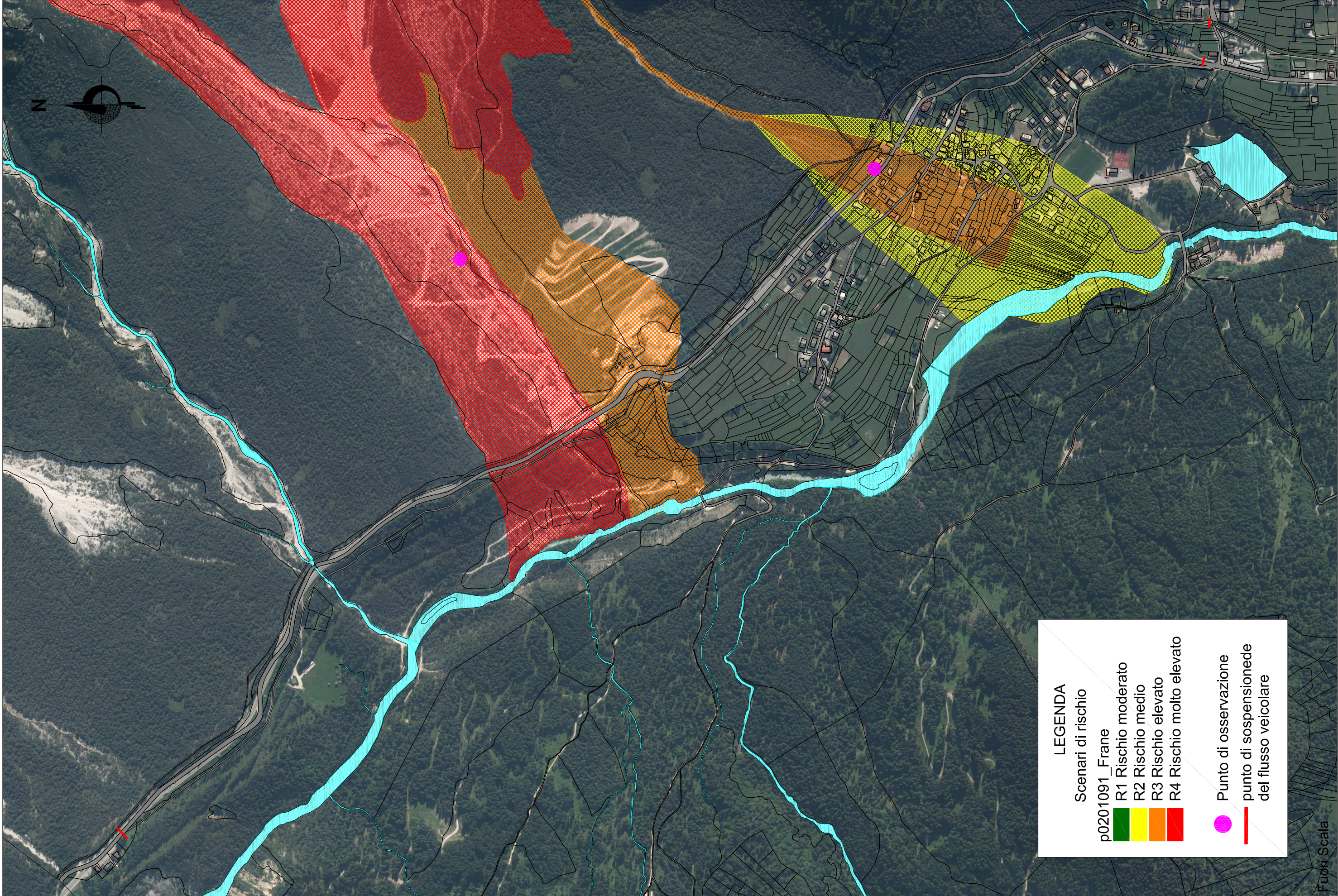
Allegato 10.A: Planimetria indicante la postazione di osservazione e i luoghi individuati per la sospensione del flusso veicolare:
