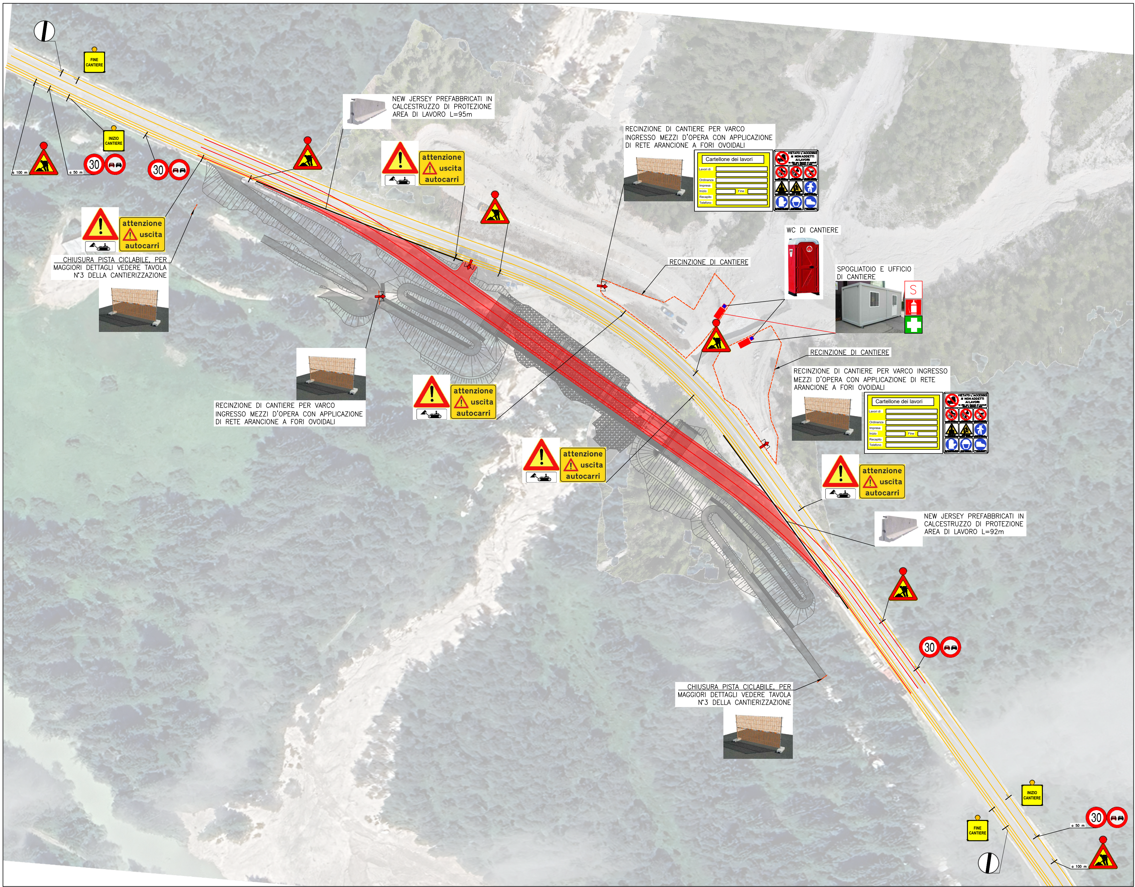
FASE 7 – ASFALTATURA E INSTALLAZIONE BARRIERE
